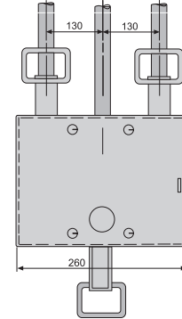
Abb. 17: Dreifachkasten-Antrieb
