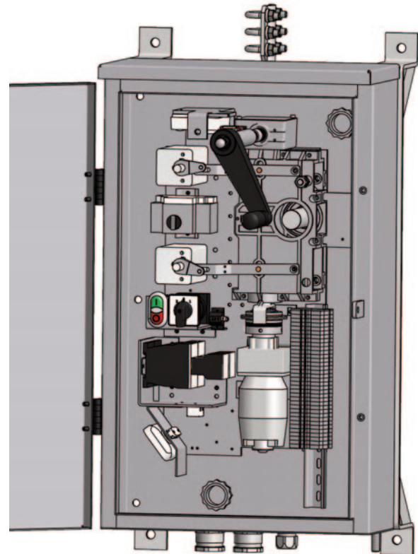
Abb. 4: z.B. Freiluft-Motorantrieb UM 90 Edelstahlgehäuse, Tür offen
