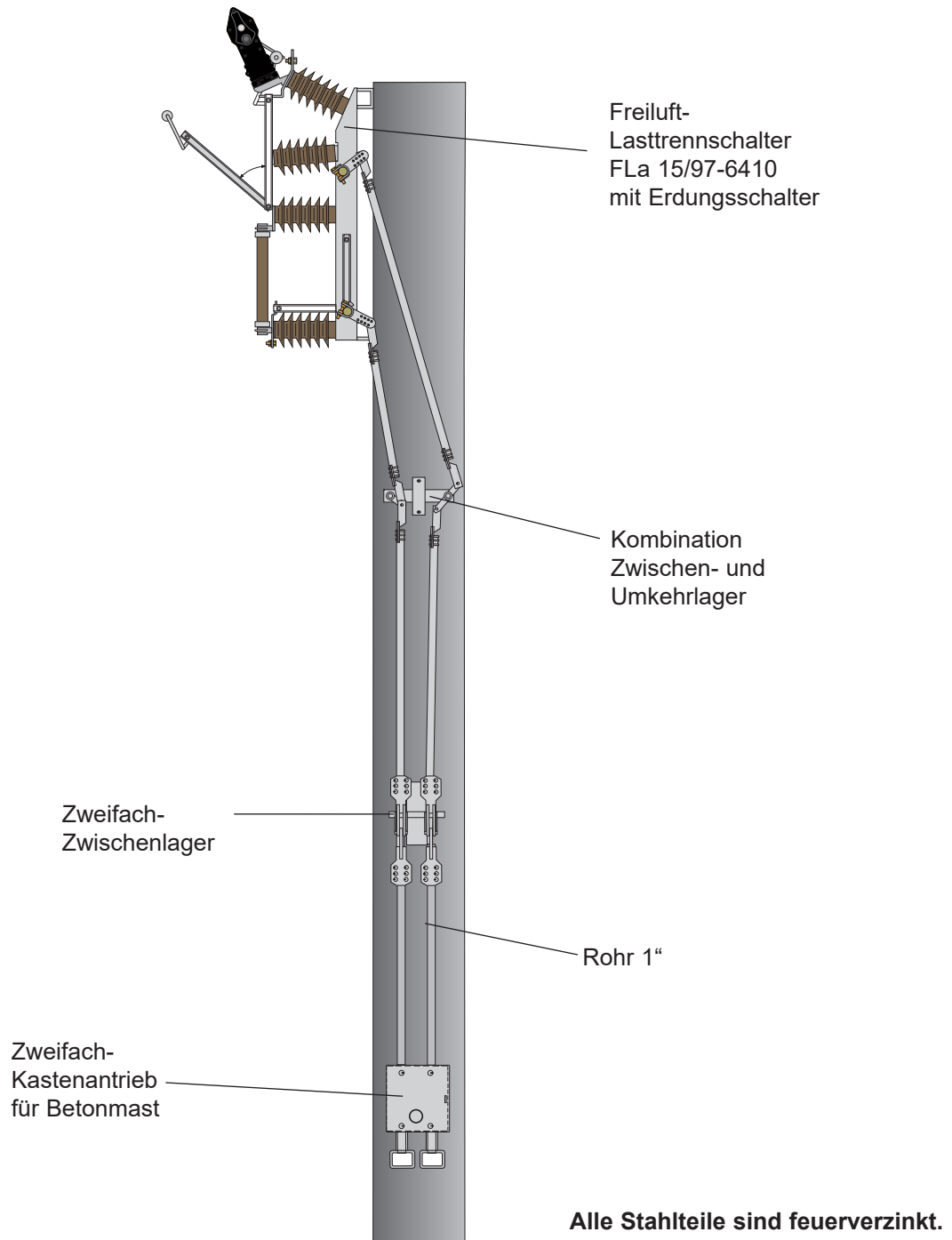
Abb. 27: Beispielhaft dargestellt Zweifach-Kastenantrieb für Betonmasten
