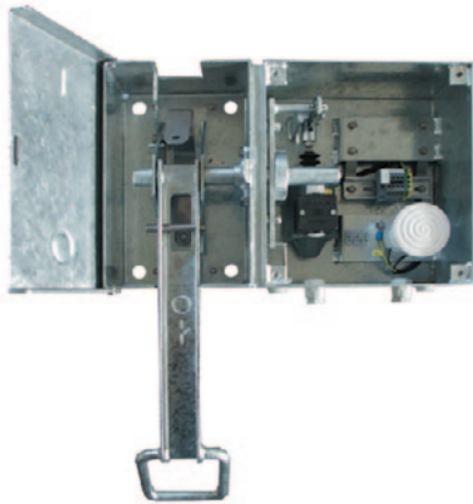
Abb. 25: Einfach-Kastenantrieb Typ 7530 mit Magnetverriegelung
