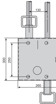
Abb. 16: Zweifachkasten-Antrieb
