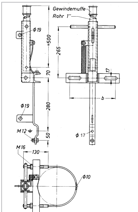
Abb. 18: L-Antrieb für Holzmast
