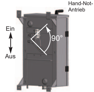
Abb. 9: Drehsinn am UM 90, Darstellung des Gehäuses aus rückseitiger Ansicht!
