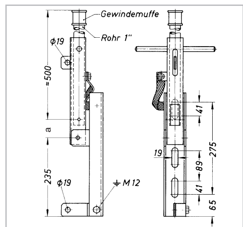
Abb. 19: L-Antrieb für Beton- bzw. Stahlmast
