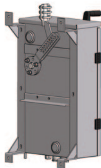
Abb. 1: Freiluft-Motorantrieb UM 90 / 350 Nm Edelstahlgehäuse
