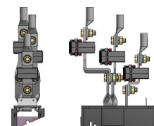
400A m. Wandlerrbau oben Z. Nr.: 117884-001 (2-84060022)
