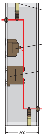
Bild 5: D 12 Meßfeld mit Strom- und Spannungswandler
