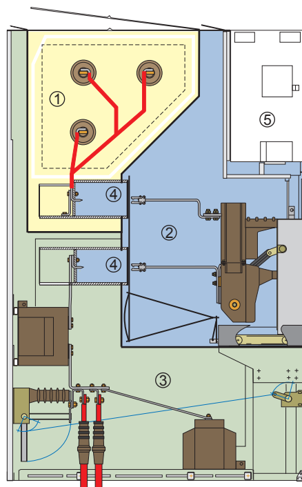
Typ E3K: 3 Kammerschottung Leistungsschalter in Trennstellung
